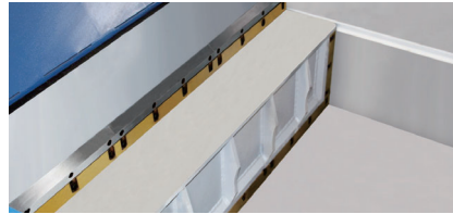
推料箱采用斜面设计，减少滞留物料。 Slanted pusher eliminates residues. 导向条寿命长，平稳推料，破碎室密封性好。 Durable guide rails ensure smooth pushing and introduces material to rotor.
